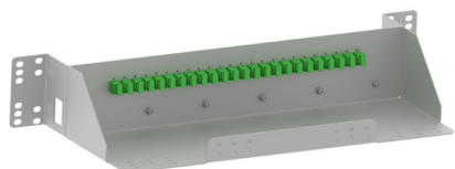
Przełącznica PS-TU-19-21/2U/24/E/SC
